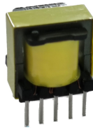
反激式变压器 Flyback Transformer
