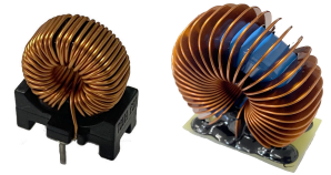
交流电感器 ACL Choke Coil
